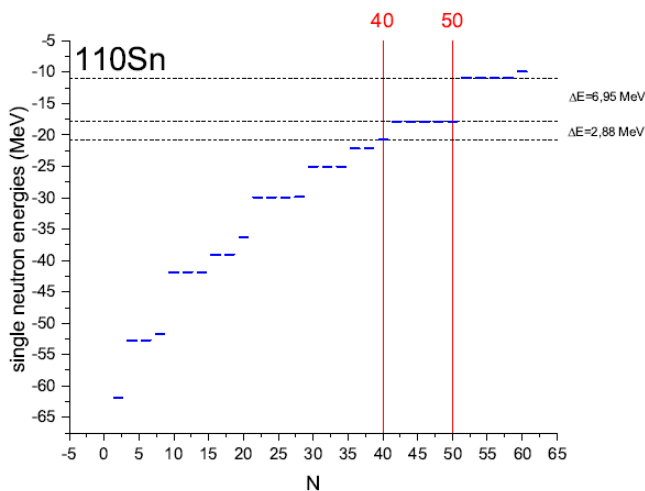
Σχήμα 5.15: Υπολογισμοί RMF για το ^{110}_{50}\text{Sn}_{60} [35]. Τα ενεργειακά χάσματα στους αριθμούς 40 και 50 είναι φανερά.
