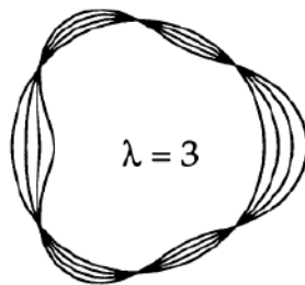
Σχήμα 1.3: Οκταπολική παραμόρφωση
