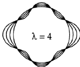
Σχήμα 1.4: Δεκαεξαπολική παραμόρφωση
