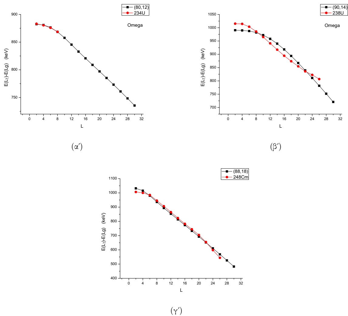
Σχήμα 6.7: Πειραματικές τιμές σε keV της ποσότητας E(L_\gamma) - E(L_g) συγκρινόμενες με τις προβλέψεις της Χαμιλτονιανής που περιέχει τον τελεστή \hat{\Omega} για ισότοπα του Ουρανίου και του Κιουρίου.
