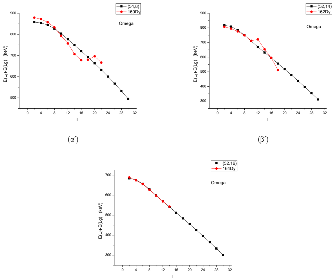
Σχήμα 6.3: Πειραματικές τιμές σε keV της ποσότητας E(L_\gamma) - E(L_g) συγκρινόμενες με τις προβλέψεις της Χαμιλτονιανής που περιέχει τον τελεστή \hat{\Omega} για ισότοπα του Δυσπροσίου.
