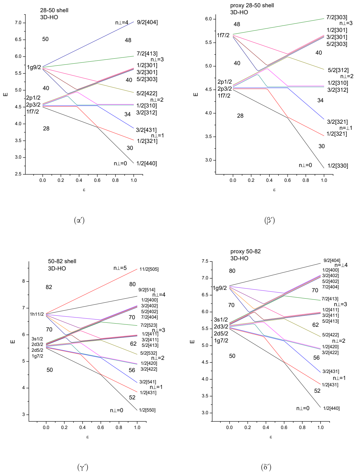
Σχήμα 5.4: Ενεργειακά διαγράμματα Nilsson για την Χαμιλτονιανή του αρμονικού ταλαντωτή για τους φλοιούς 28-50, 50-82.
